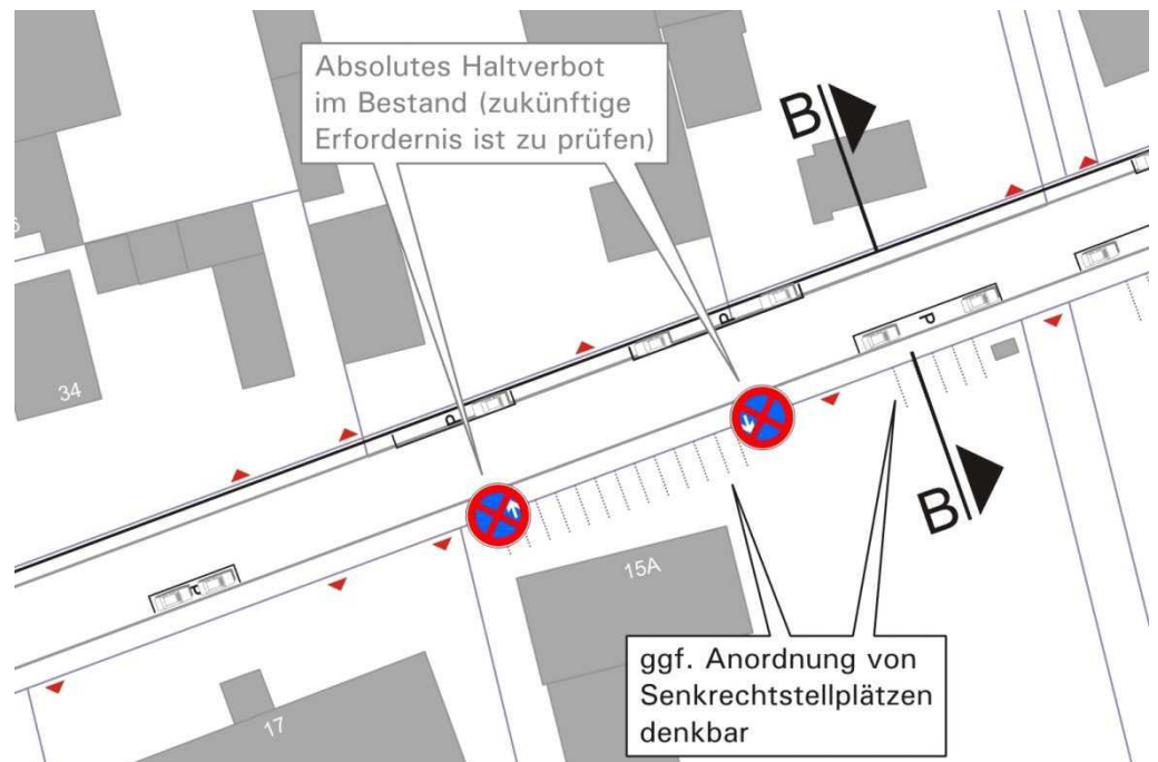
Abb. 43 Lageplanausschnitt des zentralen Bereichs (Variante 4)
