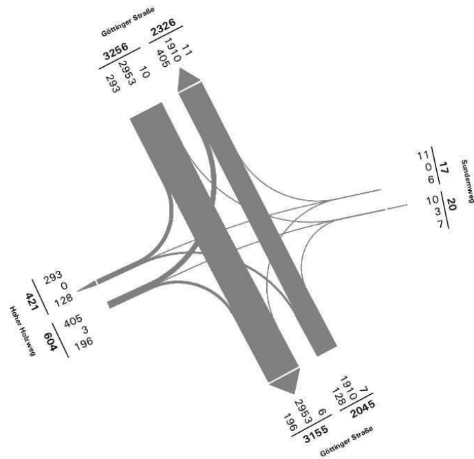
Stromplan Knotenpunkt 09: Hoher Holzweg/Göttinger Straße Zeitbereich 15:00-19:00 Uhr, Pkw, Lieferfahrzeugen und Lkw
