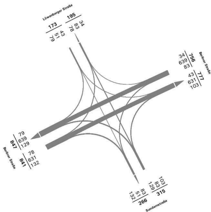
Stromplan Knotenpunkt 21: Berliner Straße/Löwenberger Straße Zeitbereich 15:00-19:00 Uhr, Pkw, Lieferfahrzeugen und Lkw
