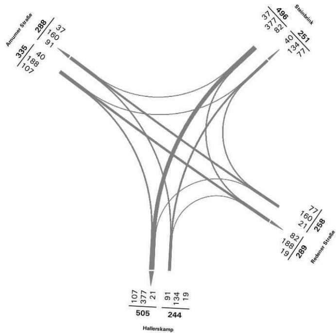
Stromplan Knotenpunkt 16: Arnumer Straße/Steinbrink Zeitbereich 15:00-19:00 Uhr, Pkw, Lieferfahrzeugen und Lkw
