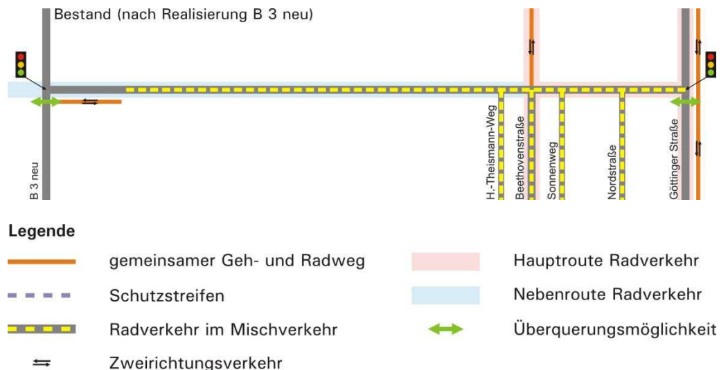
Abb. 35 Bestandssituation und Legende zum Variantenvergleich (Abb. 36)
