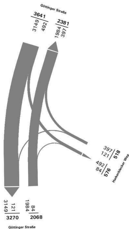
Stromplan Knotenpunkt 11: Göttinger Straße/Hakenblecker Weg Zeitbereich 15:00-19:00 Uhr, Pkw, Lieferfahrzeugen und Lkw
