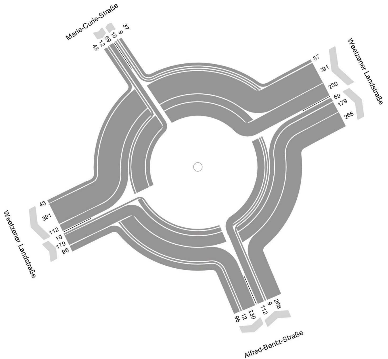
Stromplan Knotenpunkt 07: Weetzener Landstraße/Alfred-Bentz-Straße Zeitbereich Spitzenstunde 16:30 – 17:30 Uhr, Pkw, Lieferfahrzeugen und Lkw
