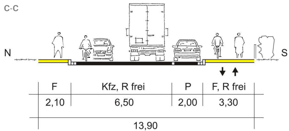
Abb. 33 Umsetzung der Variante 3 im westlichen (oben), zentralen (Mitte) und östlichen Abschnitt (unten) des Hohen Holzweges
