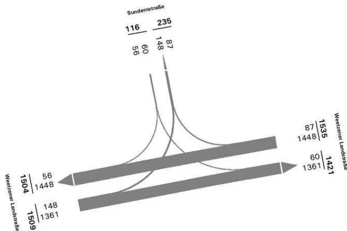
Stromplan Knotenpunkt 22: Weetzer Landstraße/Sundernstraße Zeitbereich 15:00-19:00 Uhr, Pkw, Lieferfahrzeugen und Lkw
