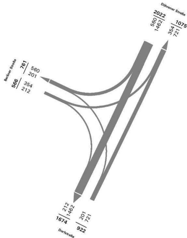
Stromplan Knotenpunkt 05: Berliner Straße/Döhrener Straße Zeitbereich 15:00-19:00 Uhr, Pkw, Lieferfahrzeugen und Lkw
