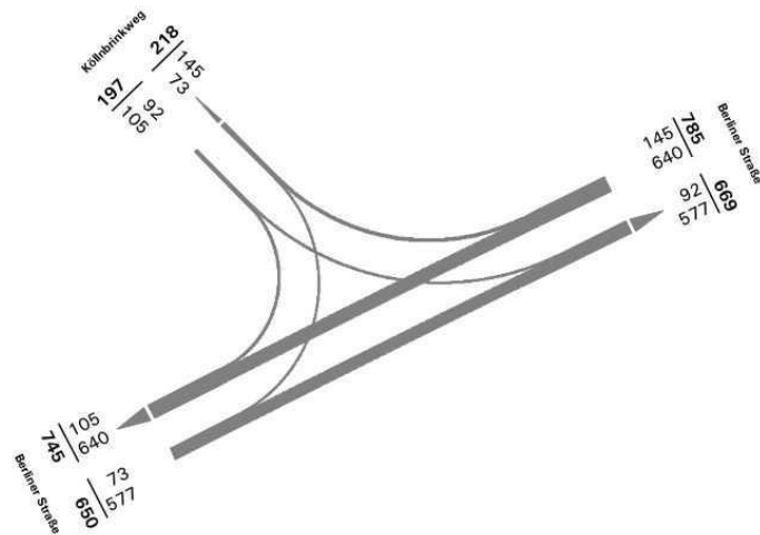
Stromplan Knotenpunkt 20: Berliner Straße/Köllnbrinkweg Zeitbereich 15:00-19:00 Uhr, Pkw, Lieferfahrzeugen und Lkw
