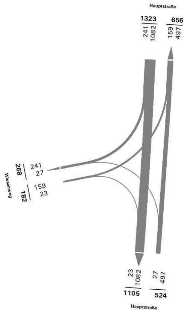
Stromplan Knotenpunkt 14: Hauptstraße/Wiesenweg Zeitbereich 15:00-19:00 Uhr, Pkw, Lieferfahrzeugen und Lkw
