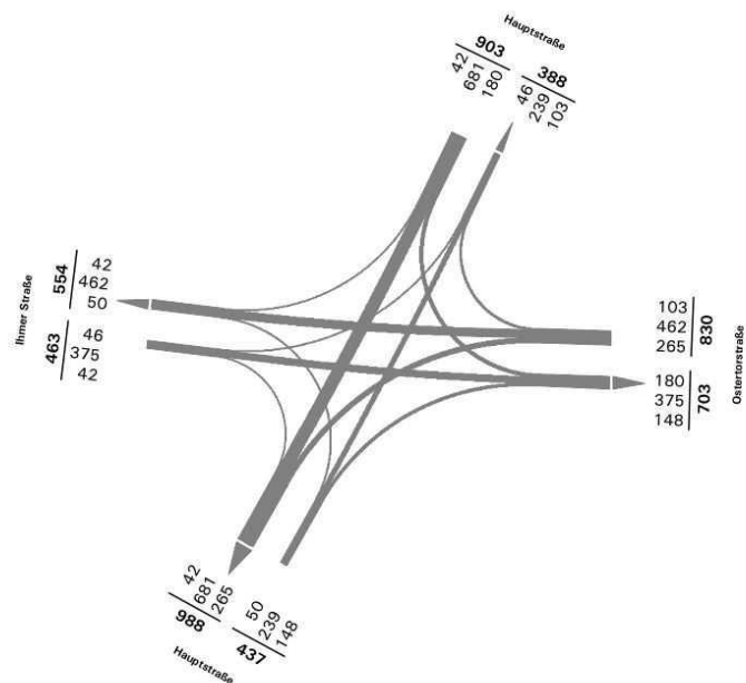
Stromplan Knotenpunkt 13: Hauptstraße/Ostertorstraße Zeitbereich 15:00-19:00 Uhr, Pkw, Lieferfahrzeugen und Lkw
