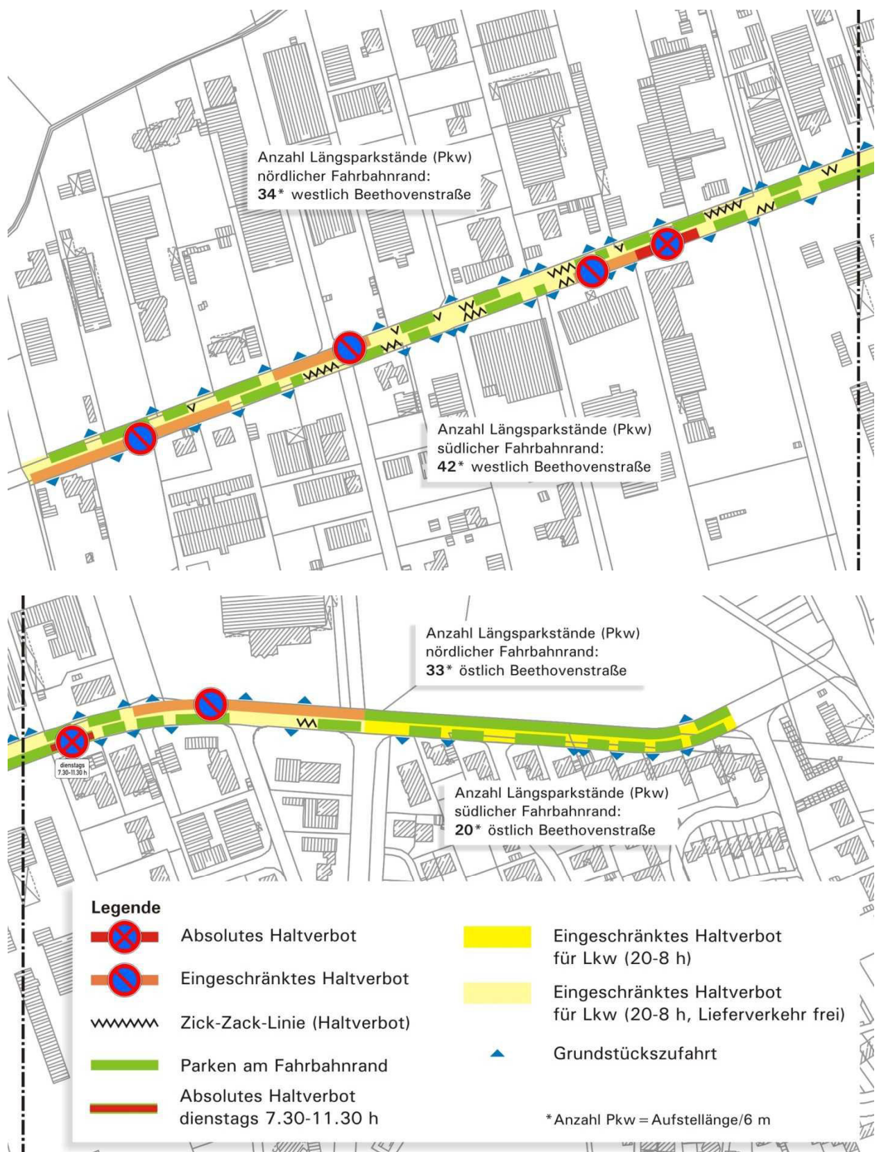
Abb. 25 Anzahl und Verortung zur Verfügung stehender Parkflächen im Straßenraum
