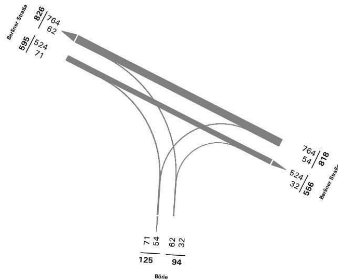
Stromplan Knotenpunkt 19: Berliner Straße/Börie Zeitbereich 15:00-19:00 Uhr, Pkw, Lieferfahrzeugen und Lkw
