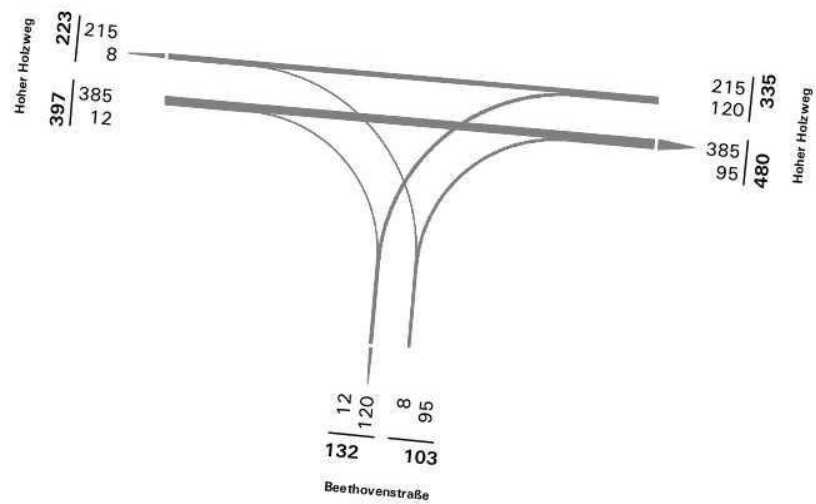
Stromplan Knotenpunkt 24: Hoher Holzweg/Beethovenstraße Zeitbereich 15:00-19:00 Uhr, Pkw, Lieferfahrzeugen und Lkw
