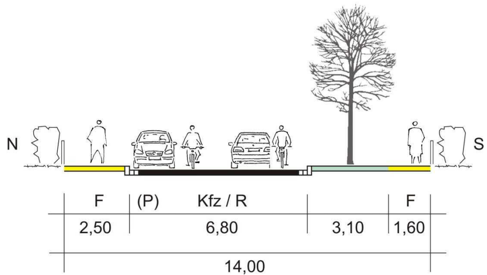
Abb. 28 Straßenraumquerschnitt A-A (westlicher Abschnitt Hoher Holzweg)
