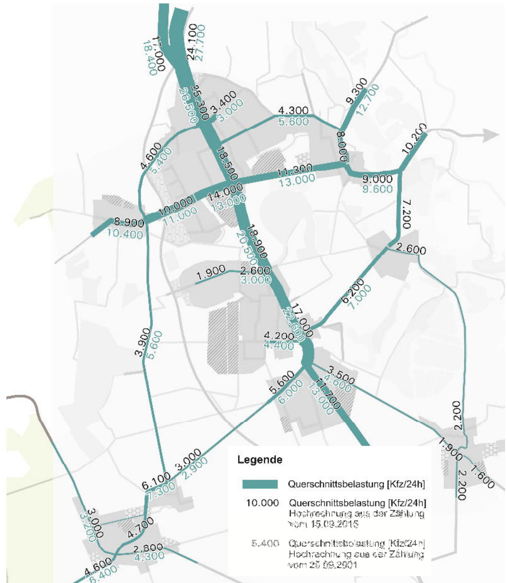
Abb. 5 Absoluter Vergleich der Querschnittsbelastungen 2001 mit 2015
