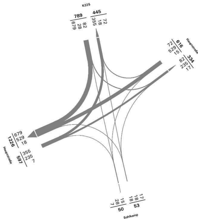
Stromplan Knotenpunkt 12: Hauptstraße/K225 Zeitbereich 15:00-19:00 Uhr, Pkw, Lieferfahrzeugen und Lkw
