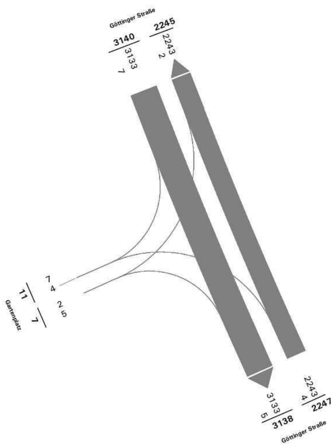
Stromplan Knotenpunkt 27: Gartenplatz Zeitbereich 15:00-19:00 Uhr, Pkw, Lieferfahrzeugen und Lkw
