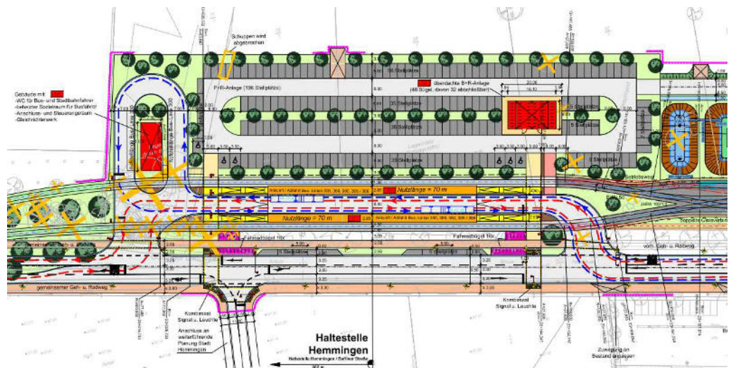
Abb. 23 Endhaltestelle Hemmingen (Quelle: Transtec, Lageplan 05/2014)
