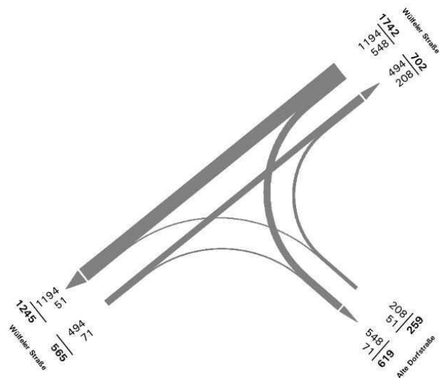
Stromplan Knotenpunkt 17: Alte Dorfstraße/Wulfeler Straße Zeitbereich 15:00-19:00 Uhr, Pkw, Lieferfahrzeugen und Lkw
