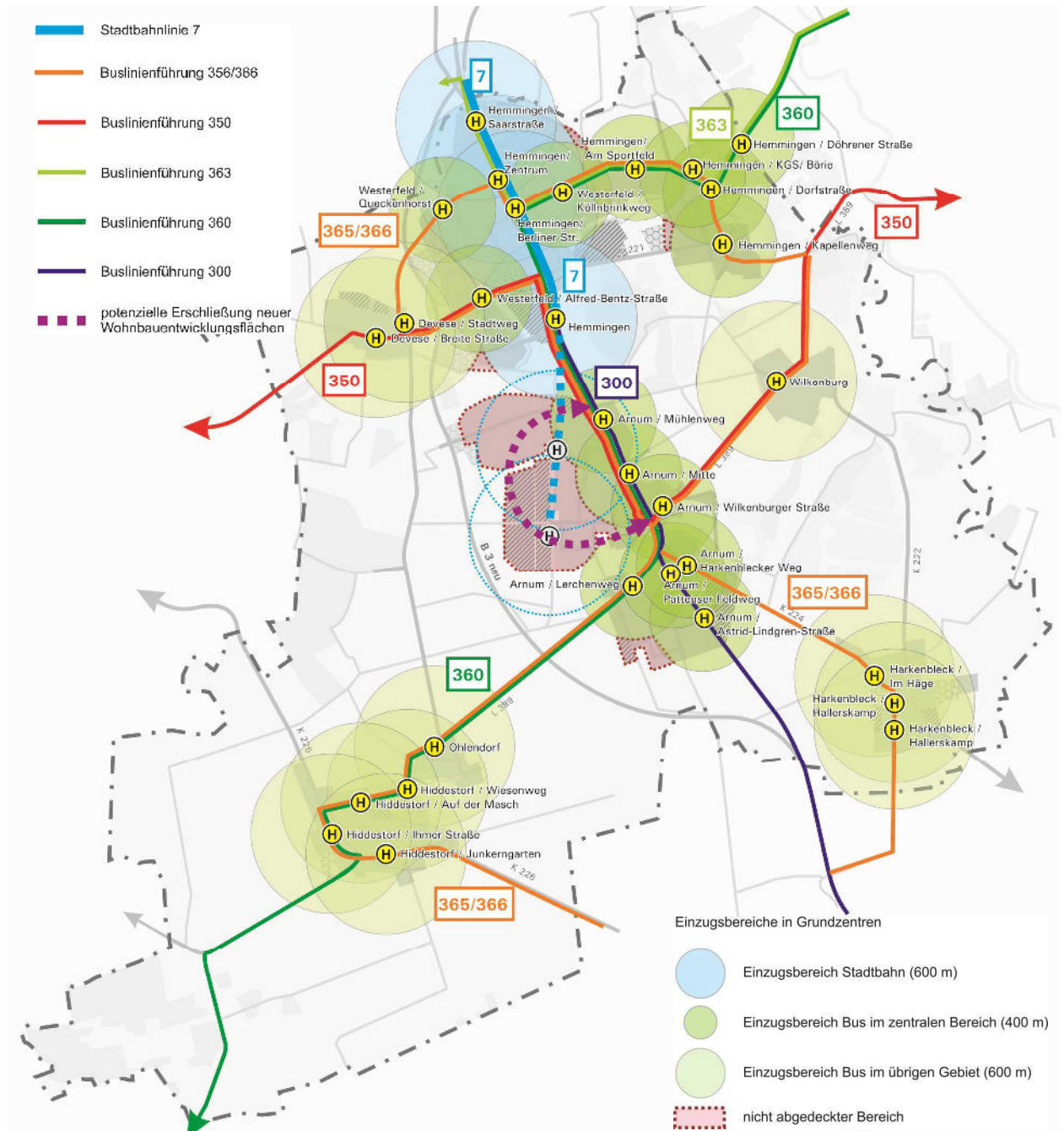
Abb. 12 ÖPNV-Linienführung nach Fertigstellung der Stadtbahnverlängerung sowie der Haltestelleneinzugsbereiche
