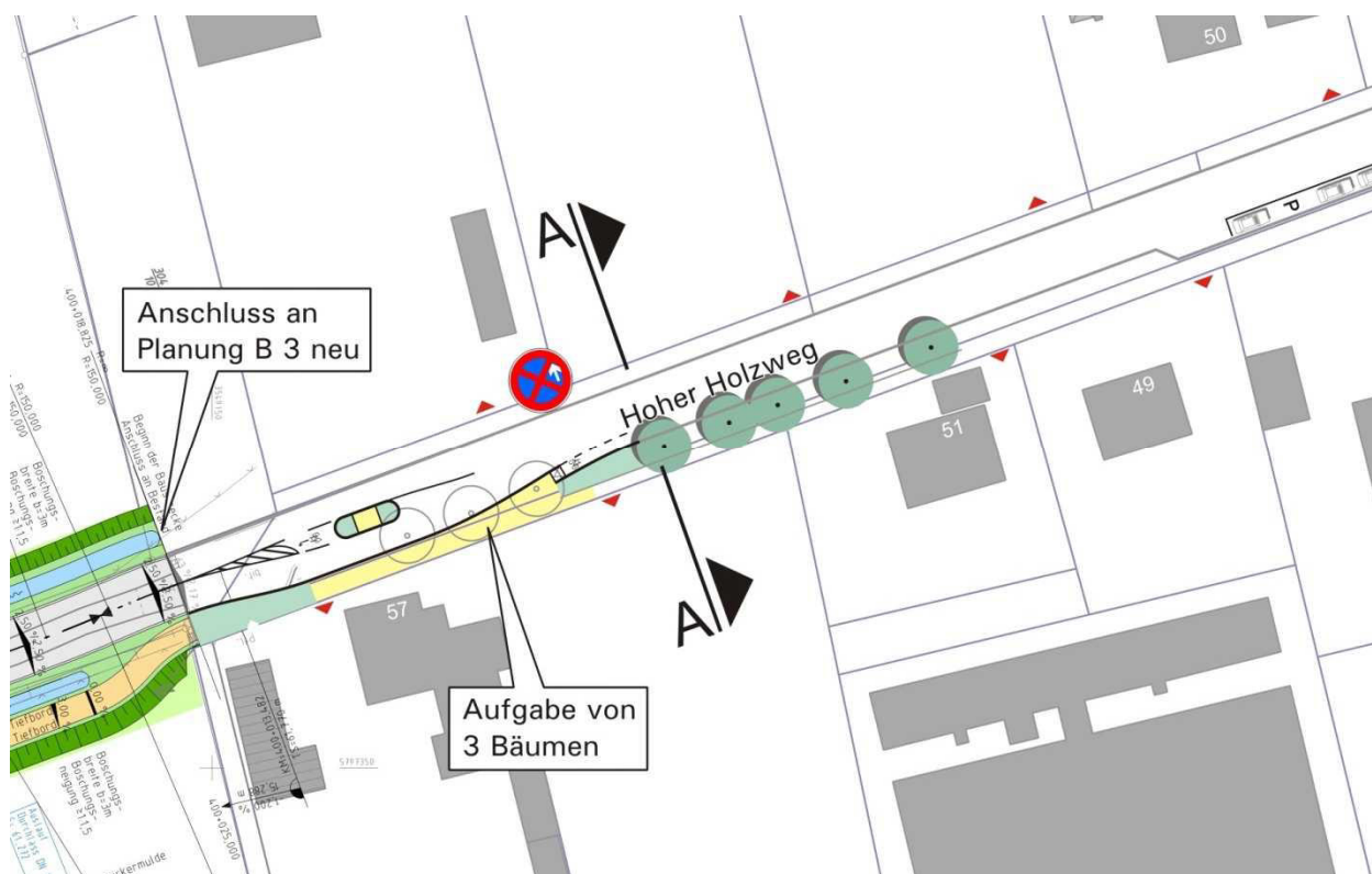
Abb. 41 Überquerungshilfe im Anschlussbereich B 3 neu (Variante 1)
