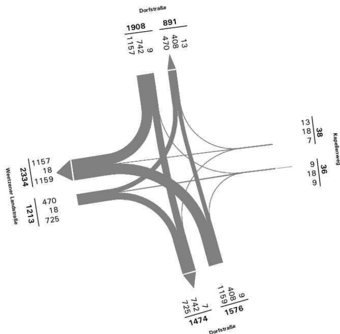
Stromplan Knotenpunkt 06: Weetzer Landstraße/Dorfstraße Zeitbereich 15:00-19:00 Uhr, Pkw, Lieferfahrzeugen und Lkw
