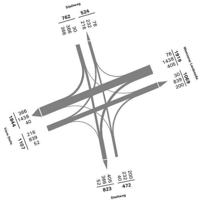
Stromplan Knotenpunkt 08: Stadtweg/Vorm Dorfe Zeitbereich 15:00-19:00 Uhr, Pkw, Lieferfahrzeugen und Lkw
