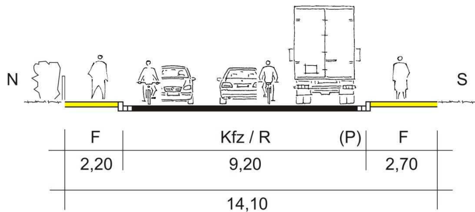
Abb. 29 Straßenraumquerschnitt B-B (zentraler Abschnitt Hoher Holzweg)
