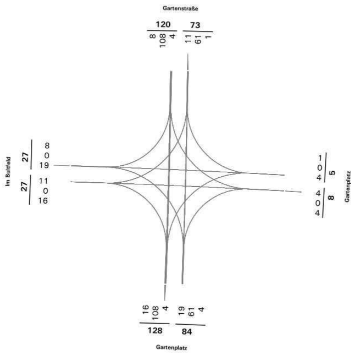
Stromplan Knotenpunkt 25: Gartenstraße Zeitbereich 15:00-19:00 Uhr, Pkw, Lieferfahrzeugen und Lkw
