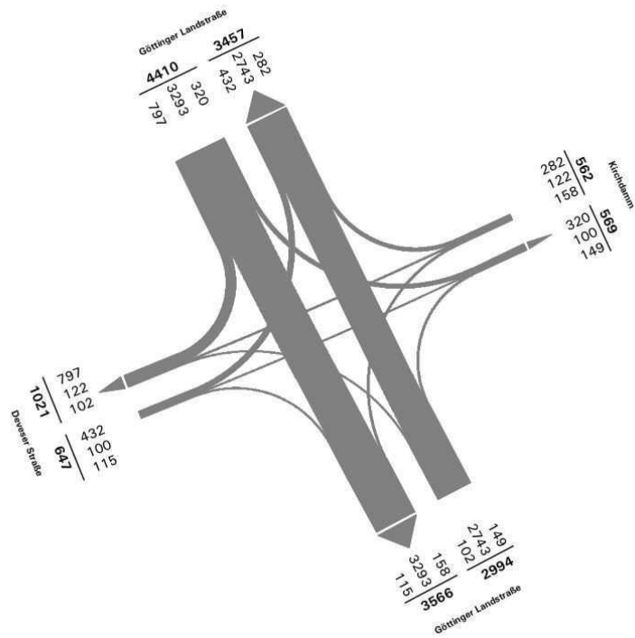
Stromplan Knotenpunkt 02: Deveser Straße Zeitbereich 15:00-19:00 Uhr, Pkw, Lieferfahrzeugen und Lkw
