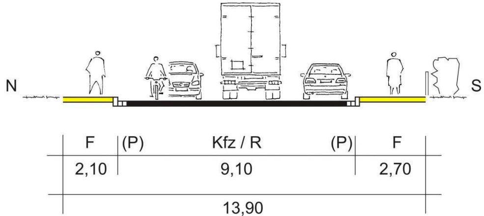
Abb. 30 Straßenraumquerschnitt C-C (östlicher Abschnitt Hoher Holzweg)
