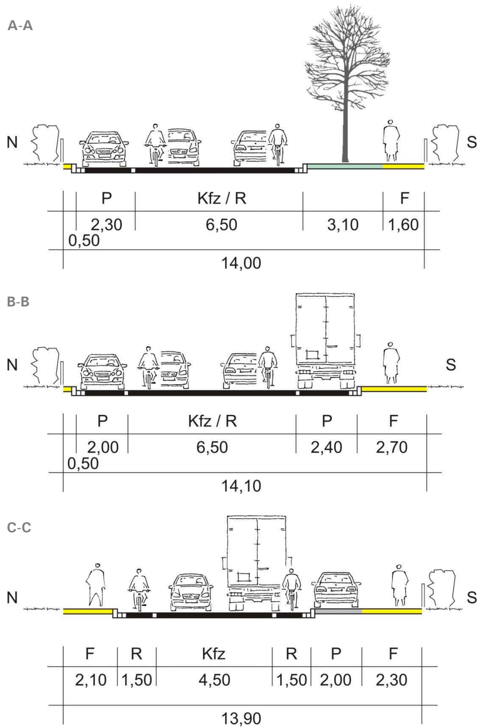
Abb. 34 Umsetzung der Variante 4 im westlichen (oben), zentralen (Mitte) und östlichen Abschnitt (unten) des Hohen Holzweges (Abschnitt C-C entspricht Variante 2)
