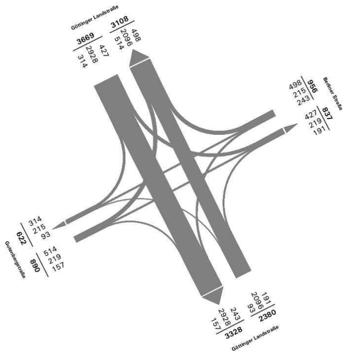
Stromplan Knotenpunkt 03: Berliner Straße Zeitbereich 15:00-19:00 Uhr, Pkw, Lieferfahrzeugen und Lkw
