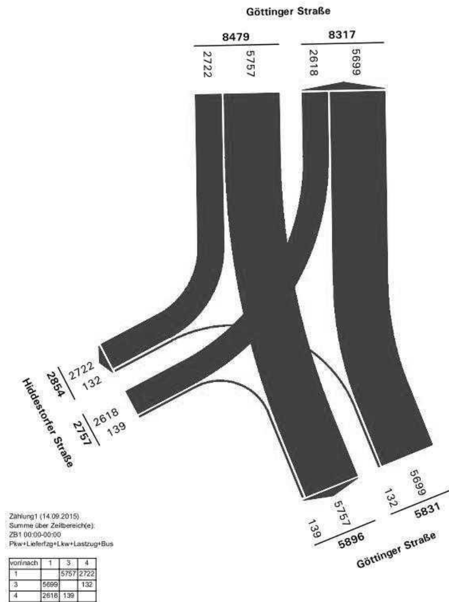
Stromplan Knotenpunkt 15: Göttinger Straße/Hiddestorfer Straße Zeitbereich 24 h, Pkw, Lieferfahrzeugen und Lkw
