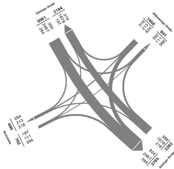
Stromplan Knotenpunkt 10: Göttinger Straße/Wilkenburger Straße Zeitbereich 15:00-19:00 Uhr, Pkw, Lieferfahrzeugen und Lkw
