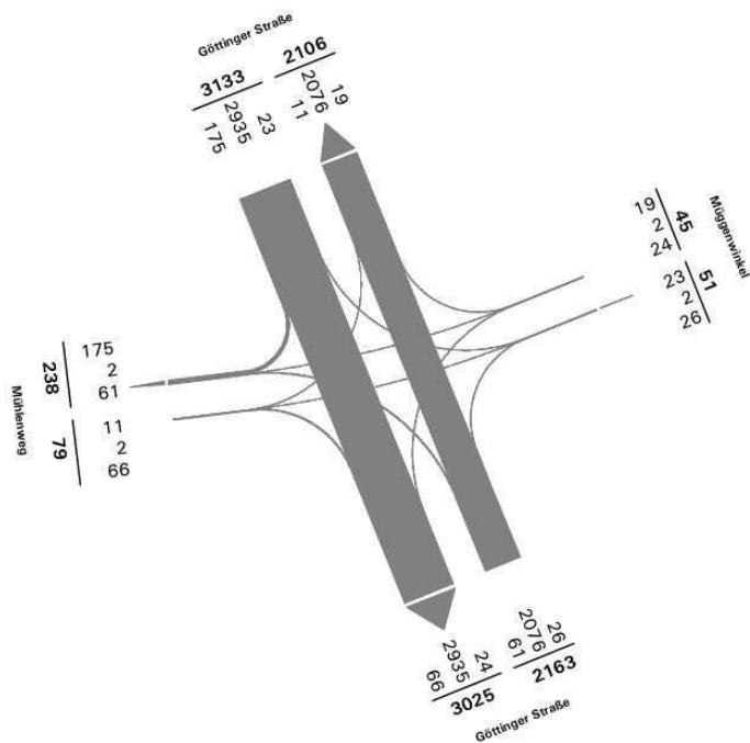
Stromplan Knotenpunkt 26: Göttinger Straße/Mühlenweg Zeitbereich 15:00-19:00 Uhr, Pkw, Lieferfahrzeugen und Lkw
