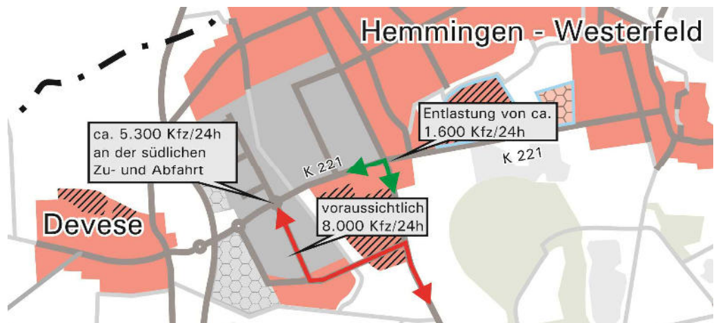
Abb. 18 Szenario 1 – Alfred-Bentz-Straße als Zubringer der neuen B3 (Zahlen basieren auf den Verkehrszählungen vom 15.09.2015 und dem von IGS erstellten Verkehrsmodell)
