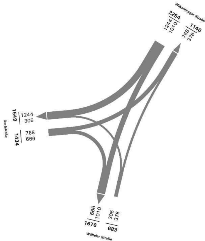
Stromplan Knotenpunkt 18: Wulfeler Straße/Wilkenburger Straße Zeitbereich 15:00-19:00 Uhr, Pkw, Lieferfahrzeugen und Lkw
