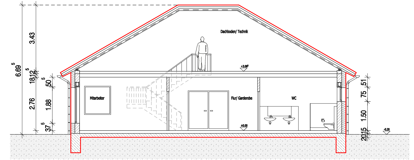
Schnitt B-B
