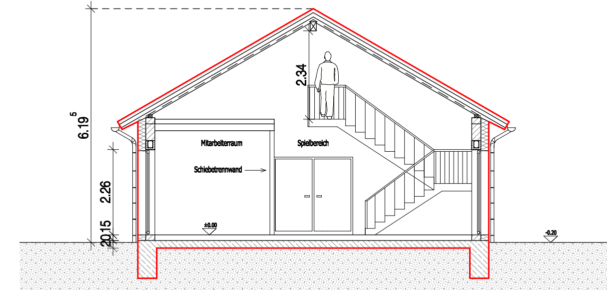
Schnitt C-C
